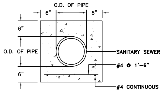
ENCASEMENT SECTION
